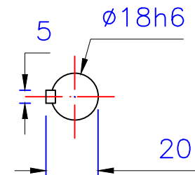
出力轴 Output shaft
